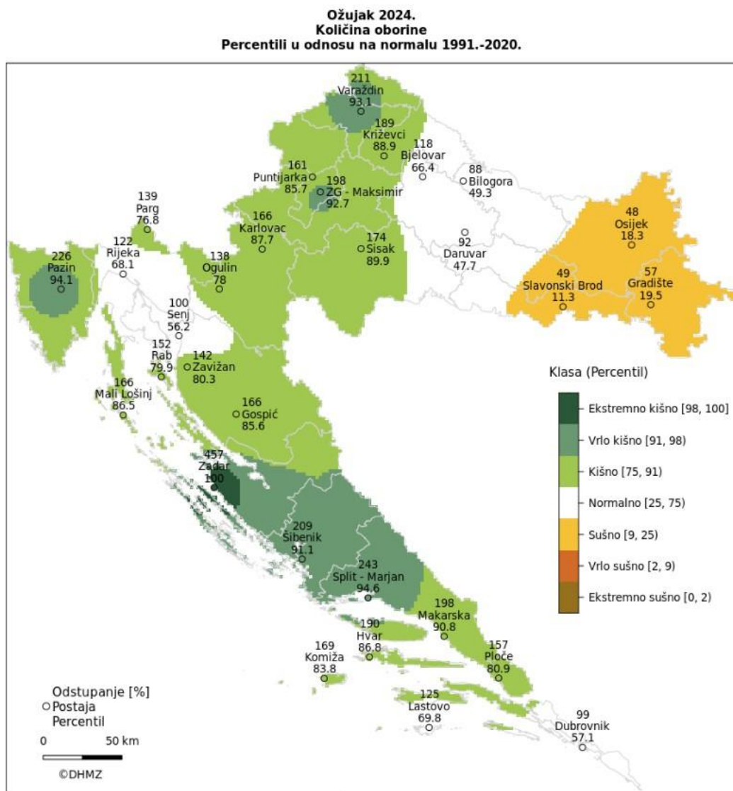
Slika 10. Odstupanje količine oborine od višegodišnjeg prosjeka za ožujak 2024. godinu
